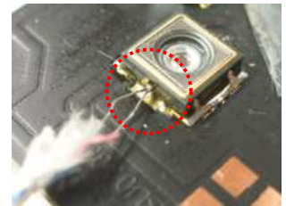
熱電対での T s 測定には、熱伝導性の高いグリスまたは接着剤をご使用下さい。
