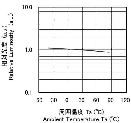
■ 周囲温度-相対光度特性 Ambient Temperature vs. Relative Luminosity
