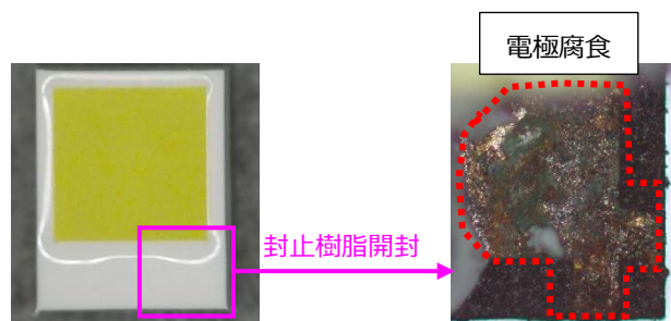
図. 塩水塗布後に点灯させた LED の外観観察結果(封止樹脂開封後に電極部を観察)
