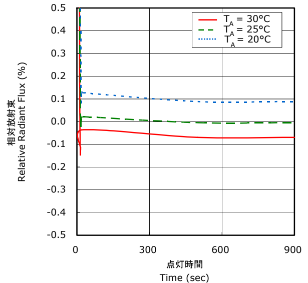
点灯時間 - 相对放射束 Relative Radiant Flux Over Time
