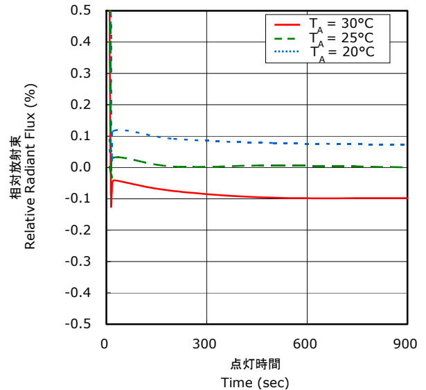
点灯時間 - 相対放射束 Relative Radiant Flux Over Time
