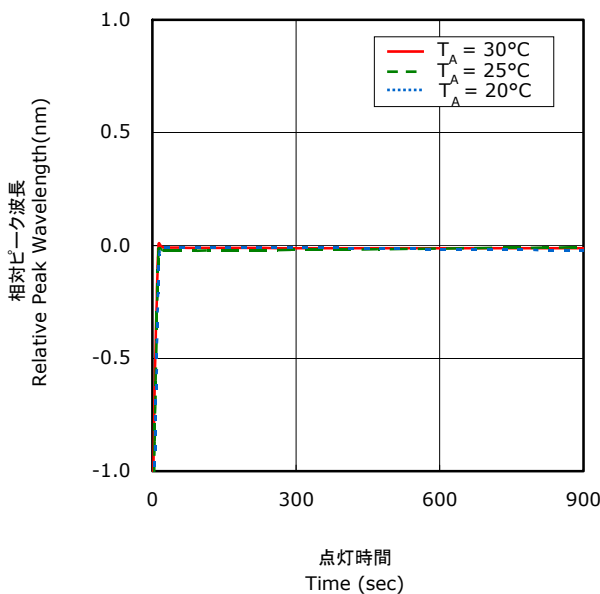
点灯時間 - 相対ピーク波長特性 Relative Peak Wavelength Over Time
