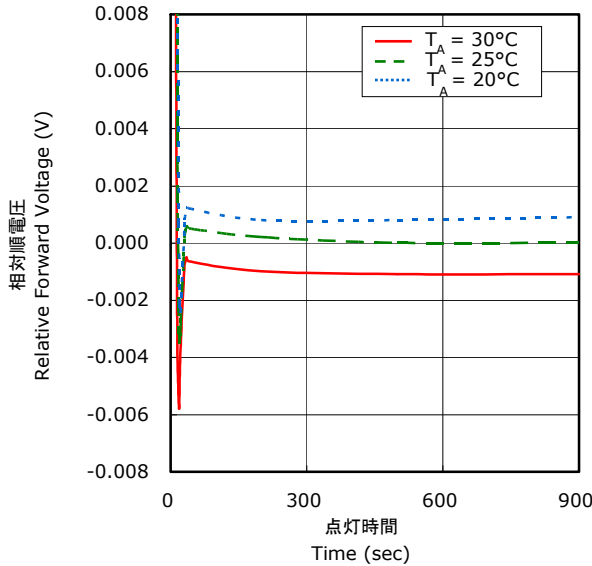
点灯時間 - 相対順電圧特性 Relative Forward Voltage Over Time
