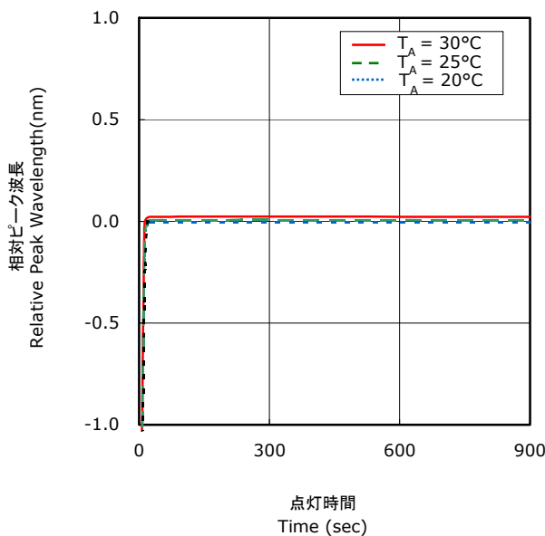
点灯時間 - 相对ピーク波長特性 Relative Peak Wavelength Over Time
